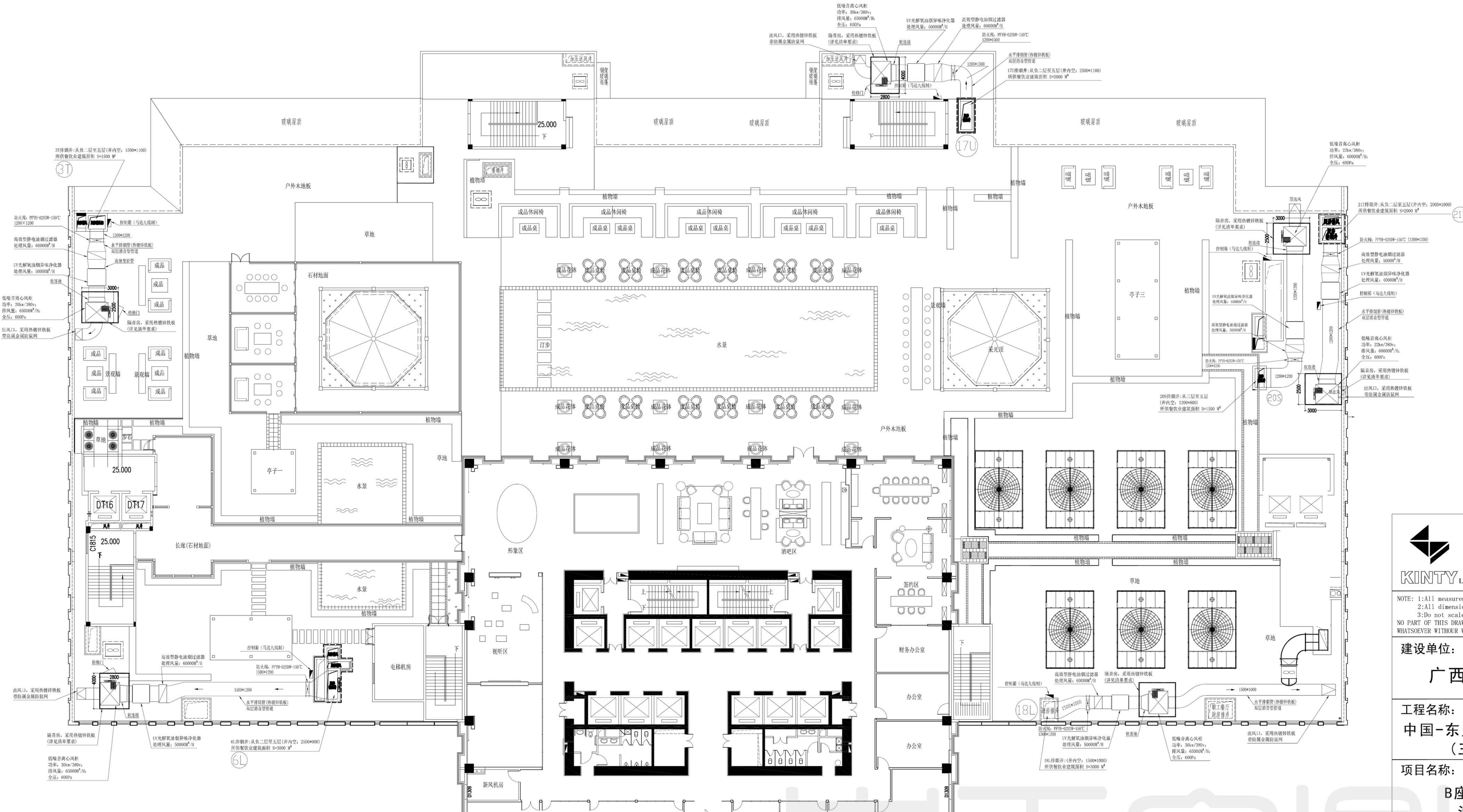
裙楼屋面设备平面图
